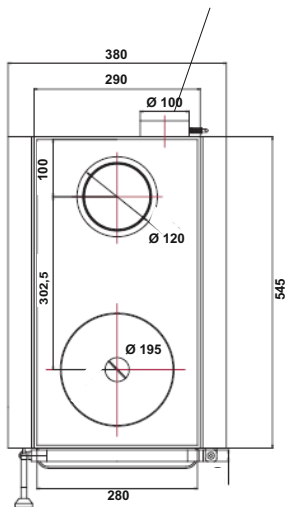
Externe luchttoevoer
