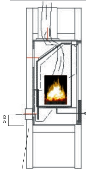
Externe luchttoevoer
